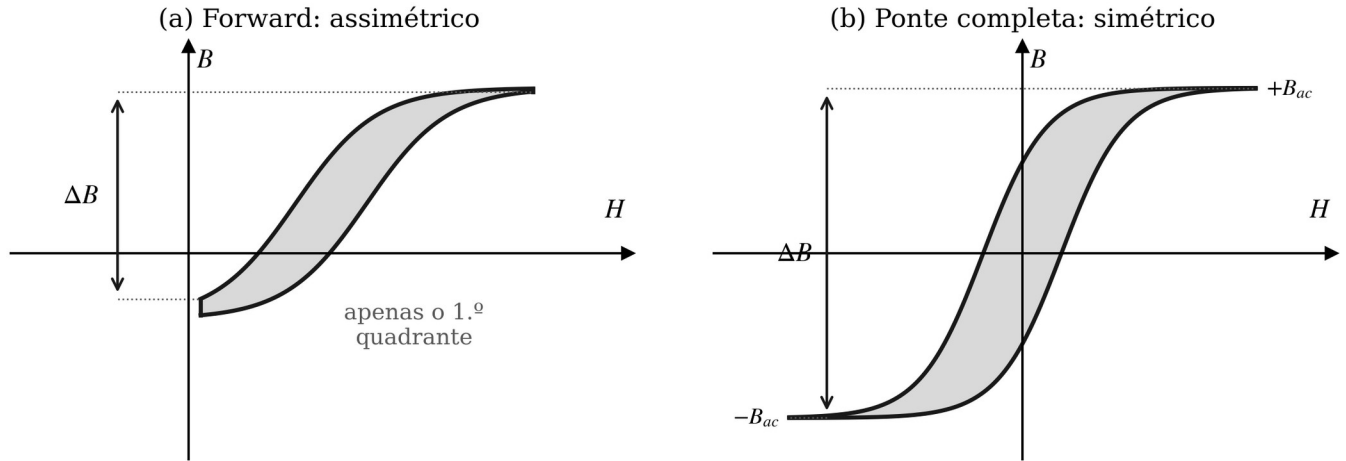
Fig. 10. Dinâmica do laço B-H nos conversores isolados. O processamento assimétrico do Forward percorre apenas o primeiro quadrante, ao passo que o processamento simétrico da ponte completa aproveita o dobro da capacidade do núcleo.
