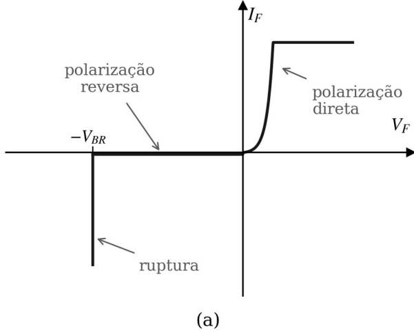
Fig. 2. Diodo de potência. (a) Característica real com as três regiões de operação. (b) Modelo linear por partes, do qual se extraem a tensão de limiar e a resistência dinâmica.
