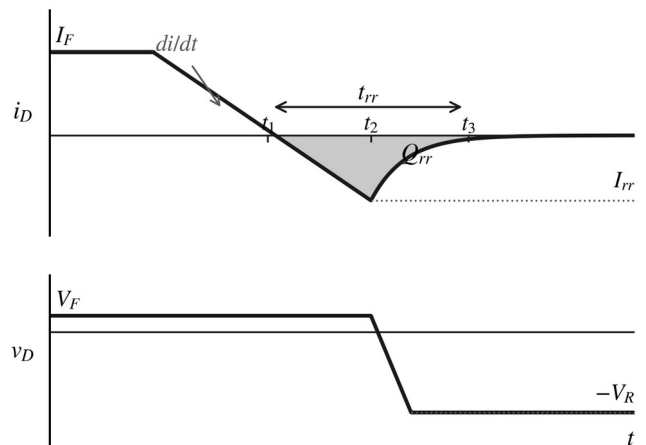
Fig. 3. Formas de onda de corrente e de tensão no bloqueio do diodo. A área hachurada é a carga de recuperação reversa, removida com a tensão reversa já aplicada.
