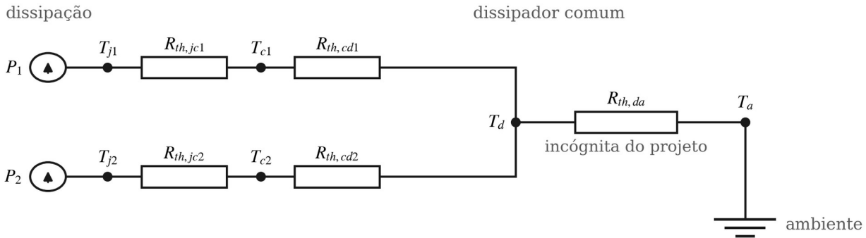
Fig. 8. Circuito térmico equivalente para dois dispositivos montados no mesmo dissipador. A potência faz o papel da corrente, a temperatura o da tensão e a resistência térmica o da resistência elétrica.
