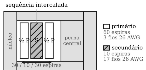
Fig. 14. Corte da janela do núcleo com a sequência de bobinagem intercalada, adotada para reduzir o efeito de proximidade e a indutância de dispersão.
