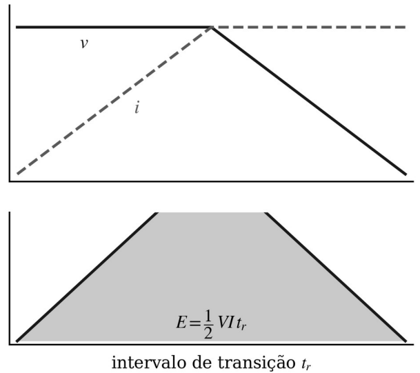
Fig. 1. Sobreposição de tensão e corrente durante a entrada em condução. Com carga resistiva as duas grandezas variam simultaneamente e a energia é um sexto do produto; com carga indutiva grampeada elas variam em sequência e a energia é a metade.
