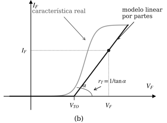
Fig. 2. Diodo de potência. (a) Característica real com as três regiões de operação. (b) Modelo linear por partes, do qual se extraem a tensão de limiar e a resistência dinâmica.
