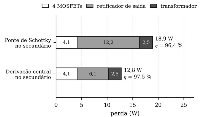
Fig. 15. Repartição das perdas do conversor completo nas duas configurações de retificador de saída. O retificador domina o balanço em ambos os casos.
